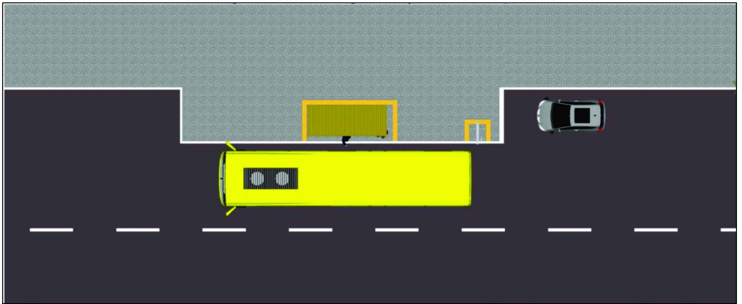
MODELO PARADA DO ÔNIBUS COM GUIA AVANÇADA VISTA TOPO SEM ESCALA FONTE: PLANO DE MOBILIDADE URBANA DE LUIZ ALVES
