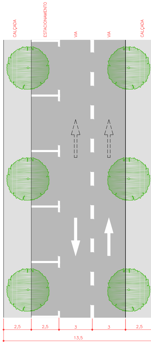
VIA LOCAL - IMPLANTAÇÃO ESCALA 1:200
