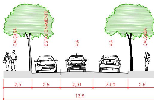
VIA LOCAL - CORTE ESQUEMÁTICO ESCALA 1:200
