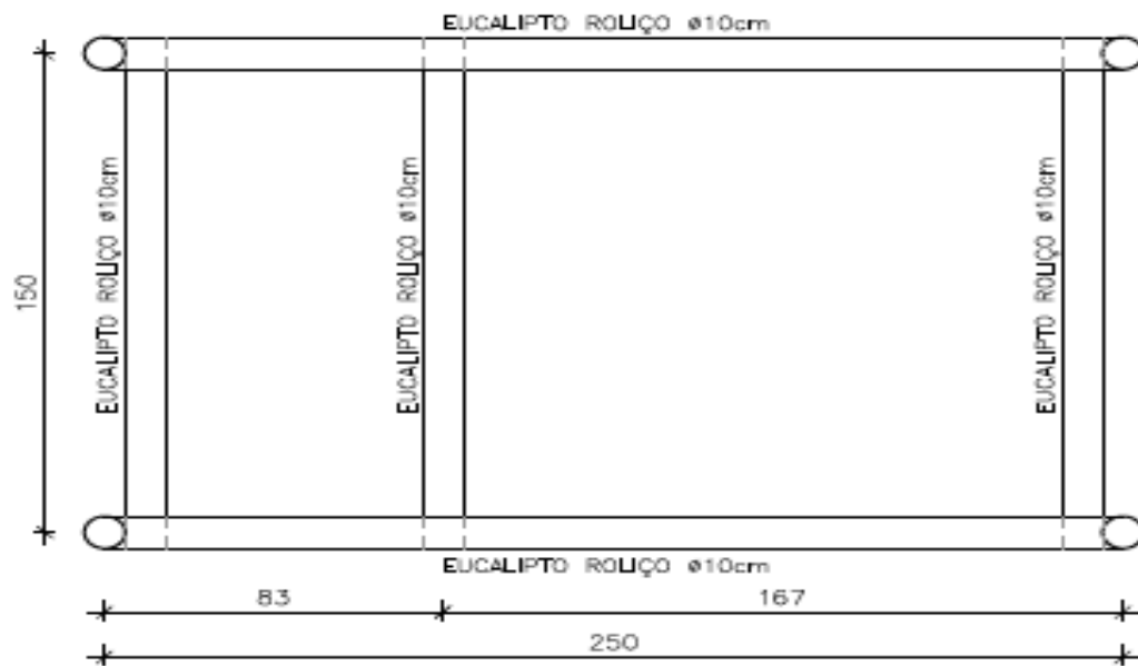
PLANTA BAIXA ESCALA 1:25
