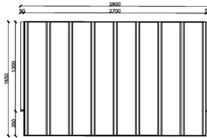
Planta de Cobertura - Abrigo de Ônibus
