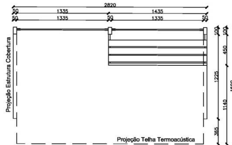
Planta Baixa - Abrigo de Ônibus
