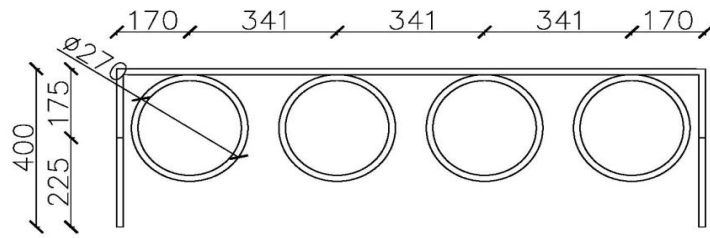
Planta Baixa - Lixeira Seletiva
