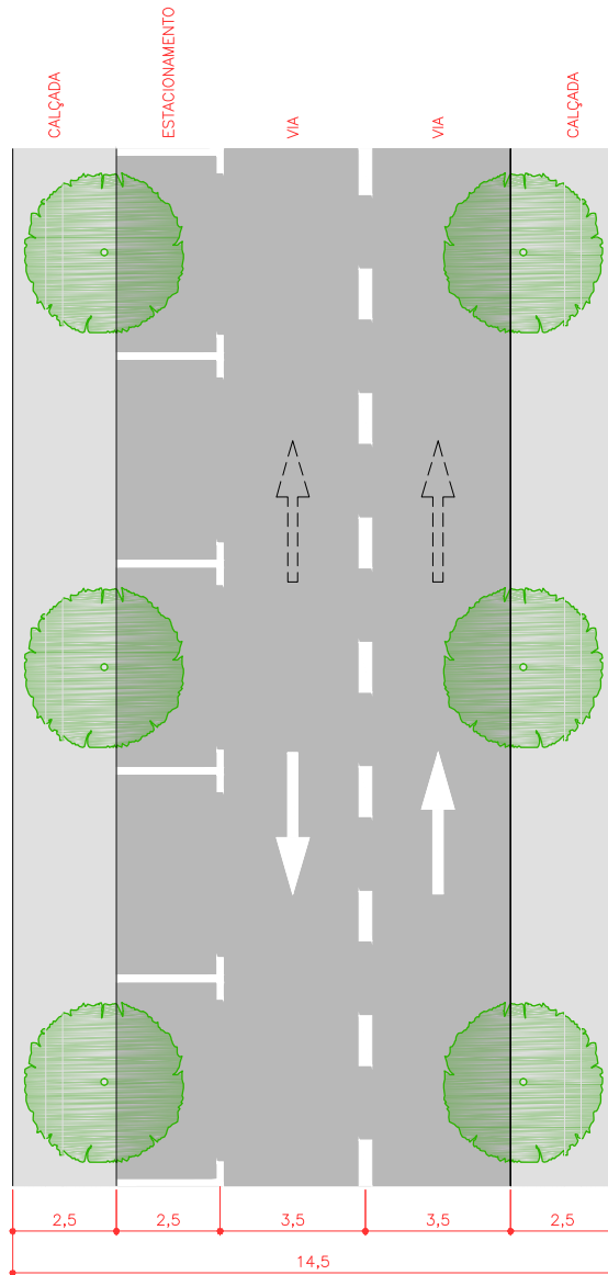
VIA COLETORA TIPO 02 – IMPLANTAÇÃO ESCALA 1:200
