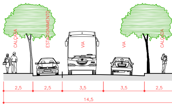
VIA COLETORA TIPO 02 – CORTE ESQUEMÁTICO ESCALA 1:200
