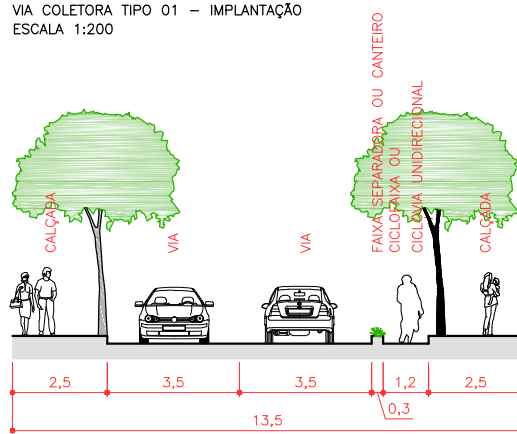
VIA COLETORA TIPO 01 - CORTE ESQUEMÁTICO ESCALA 1:200
