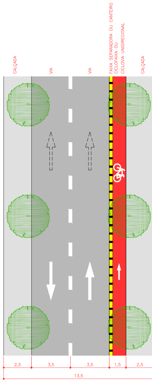
VIA COLETORA TIPO 01 - IMPLANTAÇÃO ESCALA 1:200
