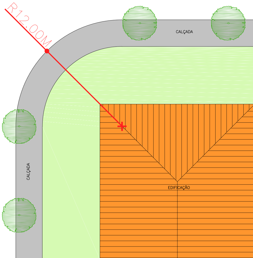
ALINHAMENTO DE MEIO FIO ALINHAMENTO DE MURO RAO DE CURVA VIA ESTRUTURAL E ARTERIAL ESCALA 1:200
